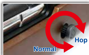
Tourner la bague hop-up pour ajuster la trajectoire des BBs. Un hop excessif peut causer le bourrage des BBs.
